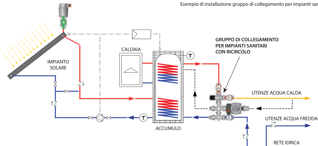
Esempio di installazione gruppo di collegamento per impianti sanitari
